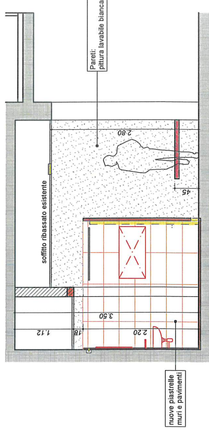
Sezione A-A
